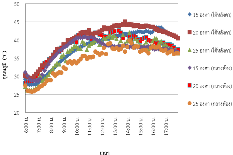
รูปที่ 5 ผลของวัสดุหลังคา (เมทัลชีส) และมูมเอียงต่อการกระจายความร้อนภายในอาคาร
